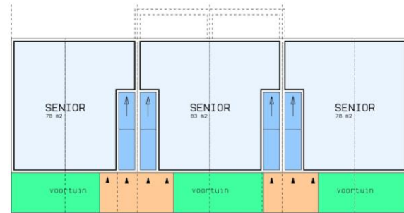
plattegrond beganegrond nieuw
